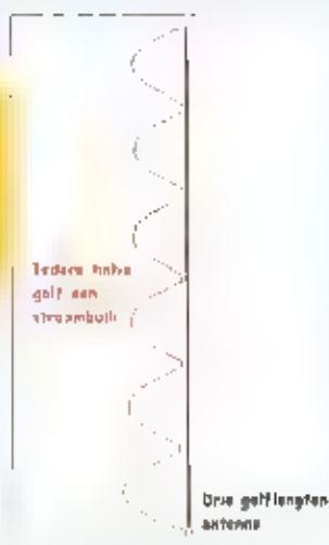
Afb. 3. Stroomverdeling in een straler van drie golf lengten lang. Het ziet er uit als zes halve golf stralers op elkaar.
